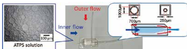
図3 マイクロ流体デバイスの同軸フローを用いるゲルフィラメントのバンドル構造体の合成。
